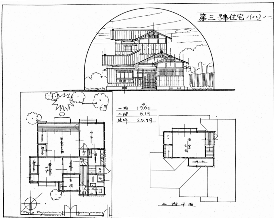
第3号住宅の(ハ)の1 立面図・平面図(No.8)
