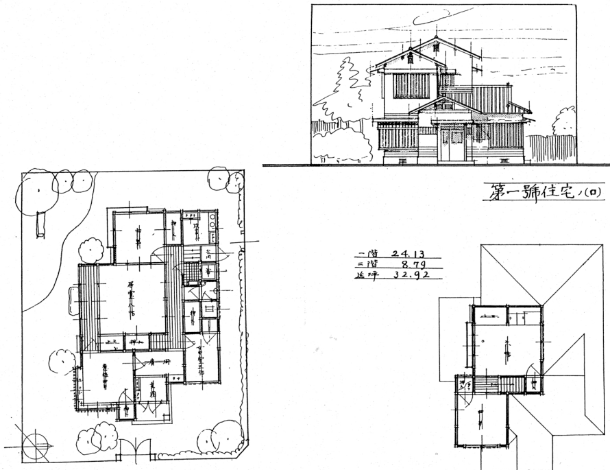
第1号住宅の(口)の立面図・平面図(No.9)
