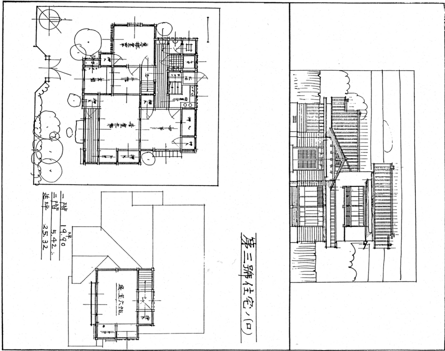
第3号住宅の(口)立面図・平面図(No5)
